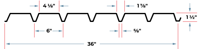
F-DECK
